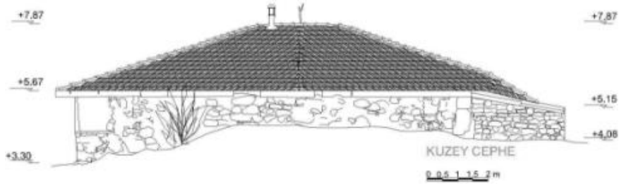
Şekil 6- Başayaş Köyü Camii planı (a), A-A Kesiti (b) ve kuzey cephesi (c) çizimleri. (Kaynak: Çizim Amir M. Efendiler, Burak Yeke ve Burcak Akyıldız'a Aittir, Ankara, 2016).
