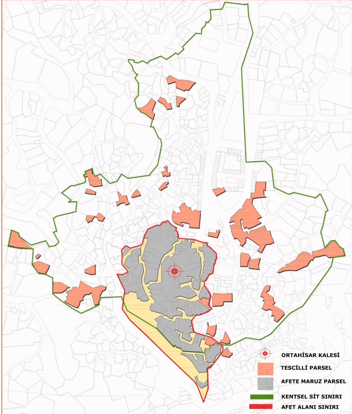
Şekil 4: Ortahisar Kalesi ve etrafında afet alanı olarak tespit edilen bölge
