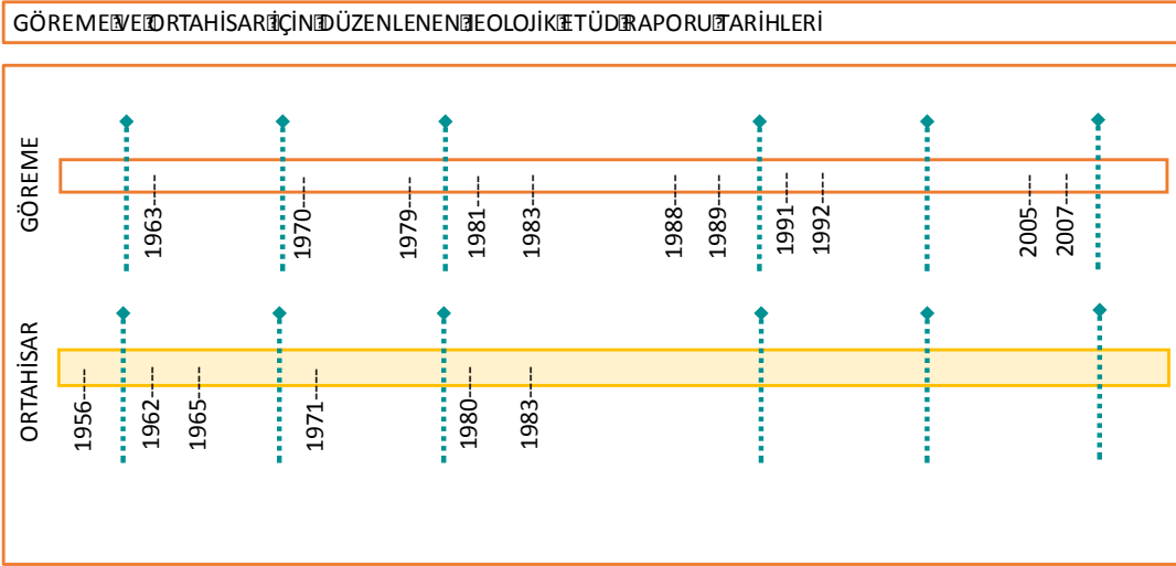
Şekil 3: Göreme ve Ortahisar için düzenlenen Jeolojik Etüd Raporu tarihleri
